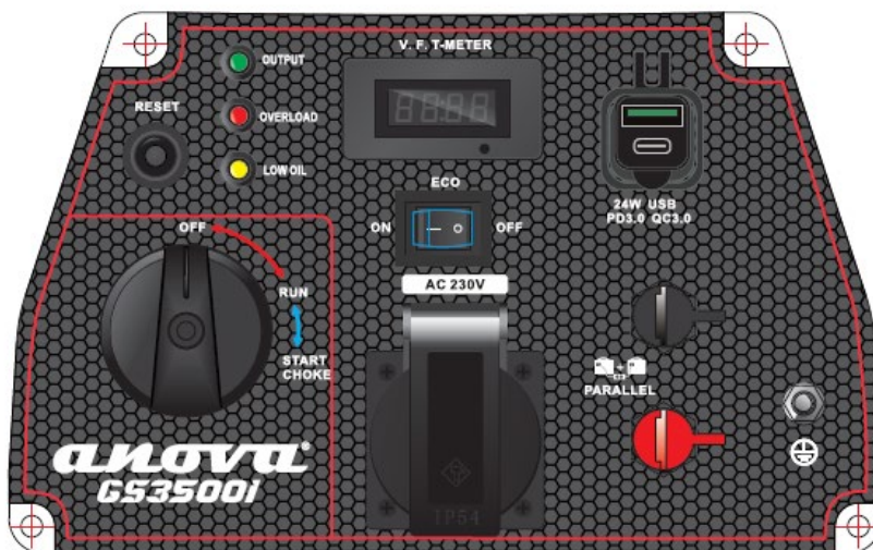
Pannello di controllo dell'unità commerciale Anova GS3500I.
