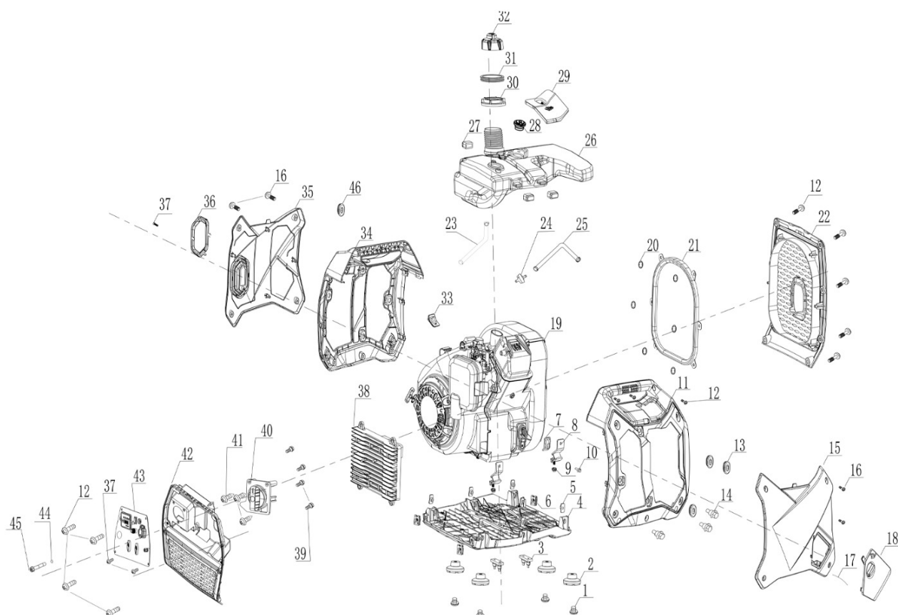
Vista generale dell'esploso del GS3500I.
