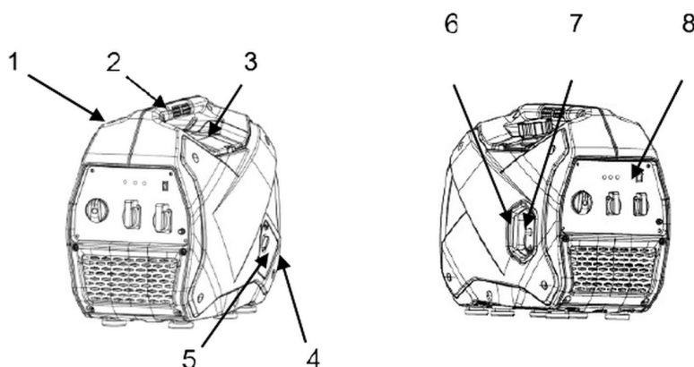
Identificazione dei componenti principali secondo il manuale del fabbricante.
