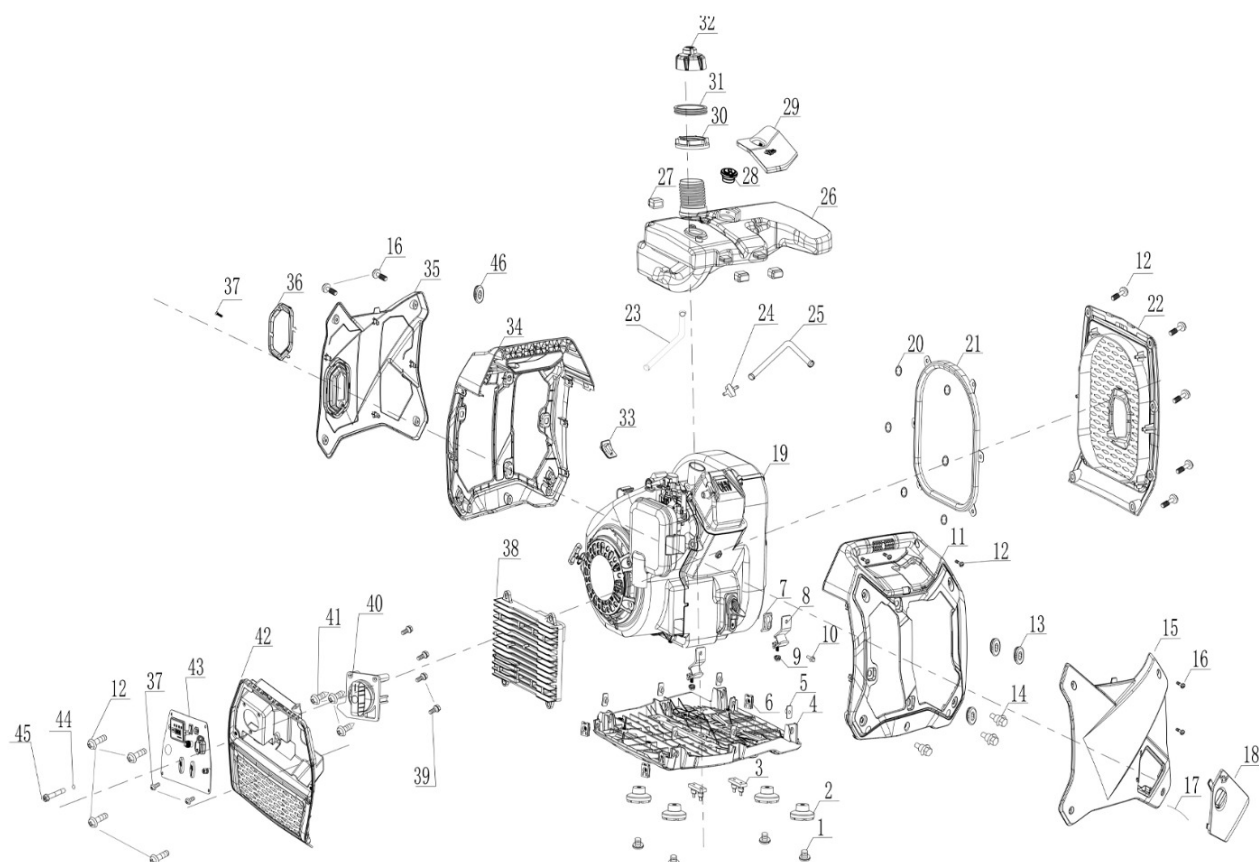
Vue générale de la vue éclatée du GS3500I.
