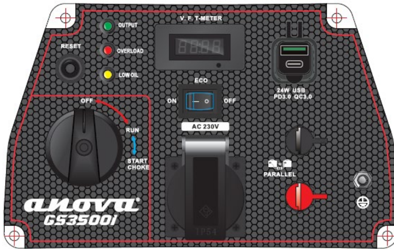
Panneau de commande de l'unité commerciale Anova GS3500I.
