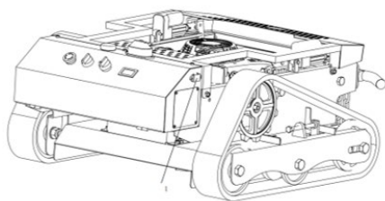
1. Presa quadrata da 24 V
